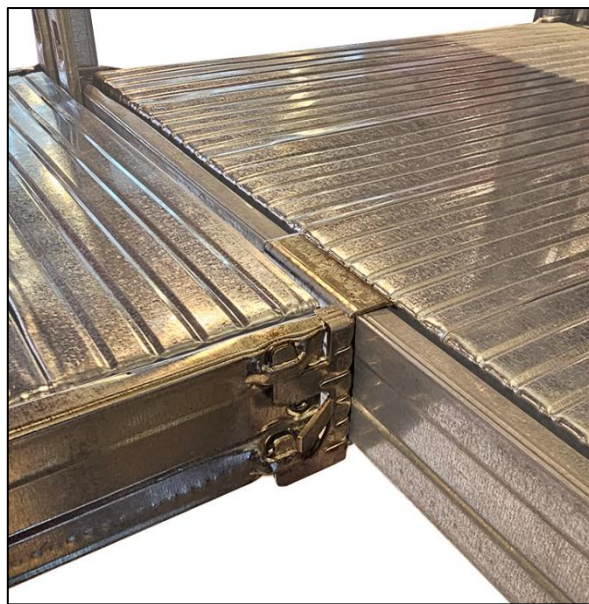
Liggerbeugel
