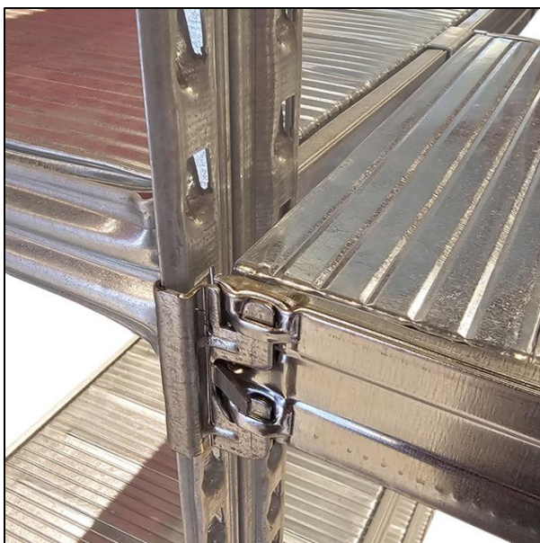
Staanderbeugel
